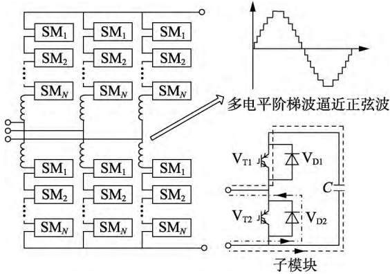
图 1 MMC 系统三相拓扑结构
