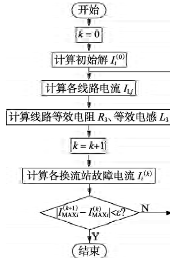
图 10 多端 MMC-HVDC 系统故障电流计算流程
