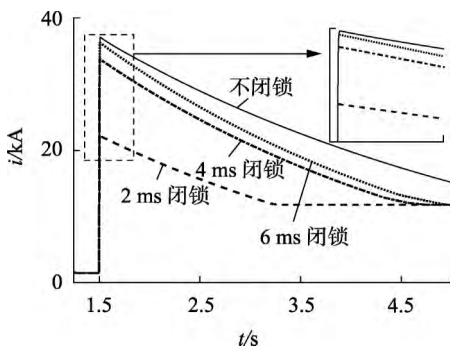
图 7 不同闭锁时间下直流线路故障电流
