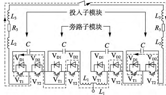
图 2 闭锁前电流通路示意图
