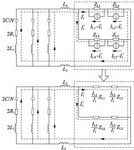
图 9 多端 MMC-HVDC 系统故障等值电路 (MMC 1 )
