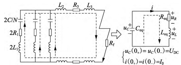
图 3 闭锁前故障等值电路及其初始条件
