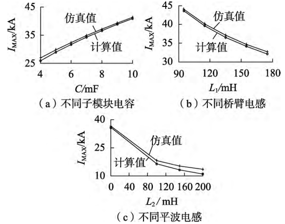
图4 不同一次系统参数下直流线路故障电流峰值
