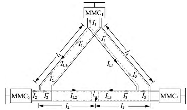
图 8 并联型三端 MMC-HVDC 系统示意图
