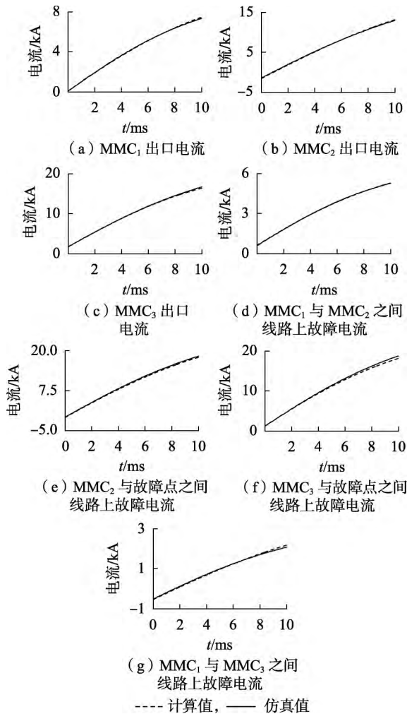
图 11 仿真结果和计算结果对比
