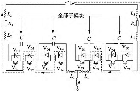
图 6 闭锁后电流通路示意图
