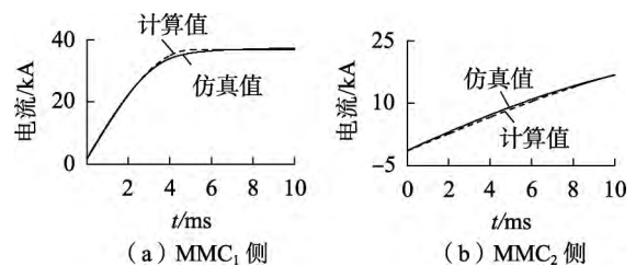
图5 线路故障电流仿真结果和计算结果对比
