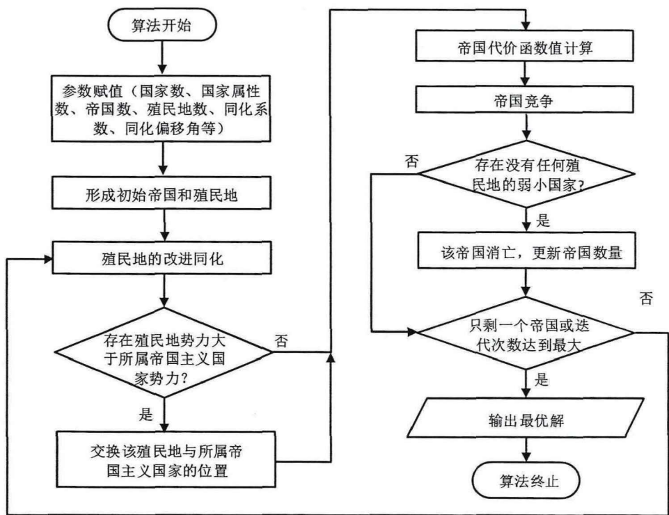
图 5-2 帝国竞争算法
