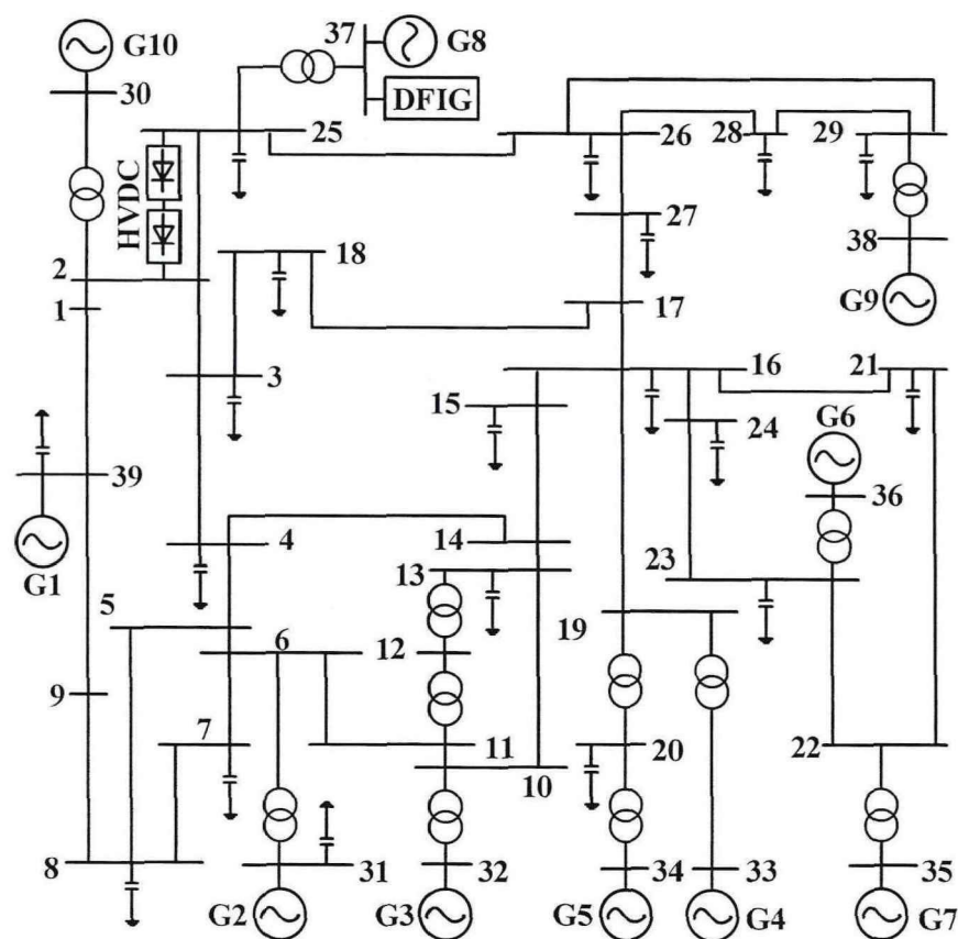
图 5-12 修改后的 10 机 39 节点系统
